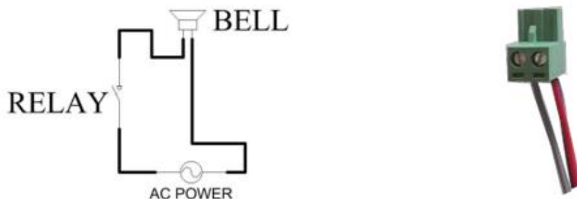
Рисунок 20 - Схема подключения сигнала
